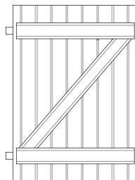
Volet à barres et écharpes
