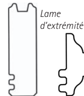
Couvre-joint pour Lame d'extrémité
