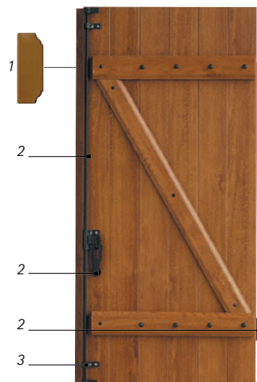
Exemple : volet avec barres et écharpes
